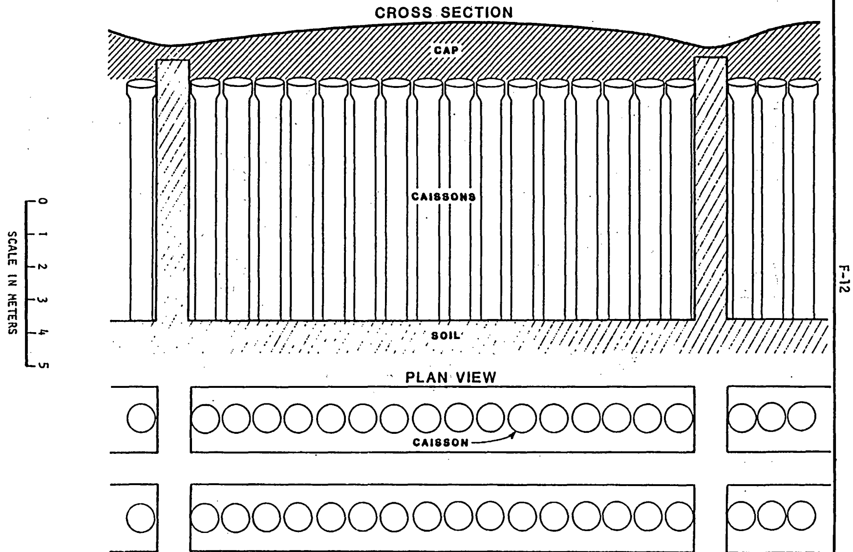
Figure F.2 Caisson Trench Disposal
