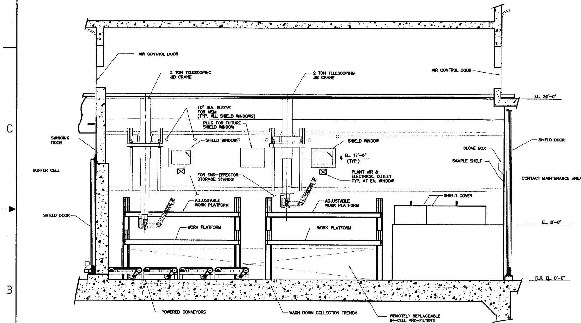
SECTION A-A
