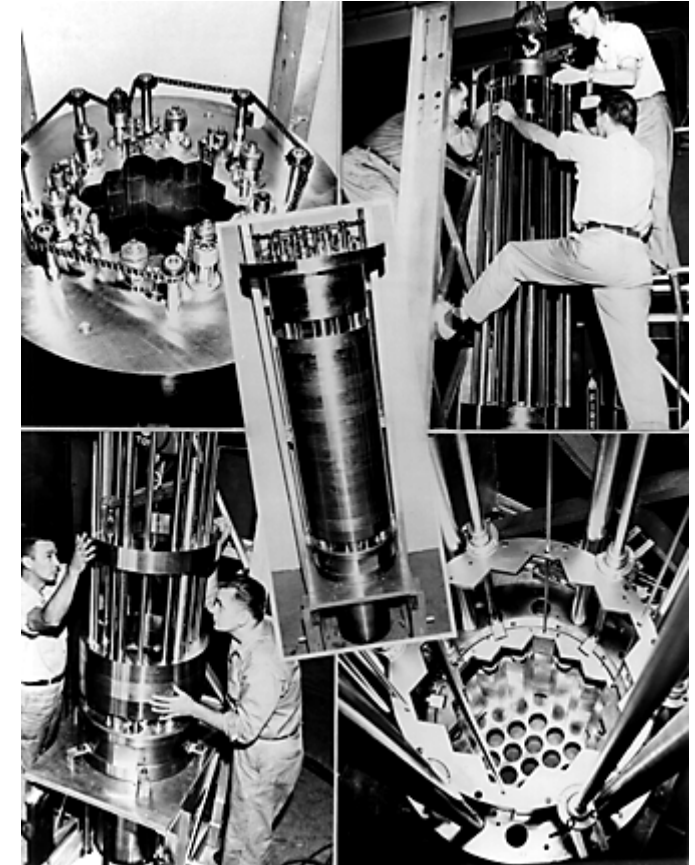
Fermi Unit 1
