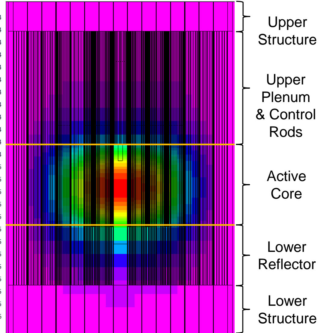
Total Flux (Linear Scale)
