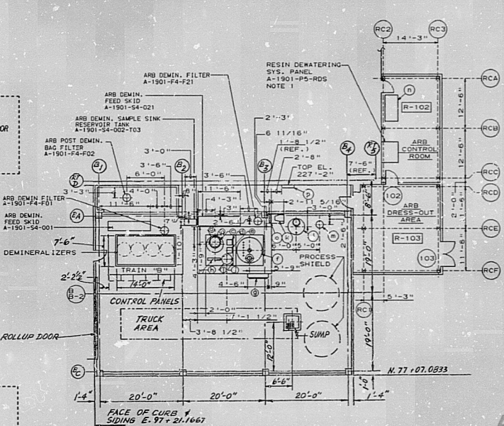
ALTERNATE RADWASTE BLDG. SCALE = N.T.S.
