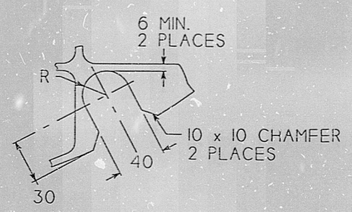
DETAIL E SCALE: 1/2
