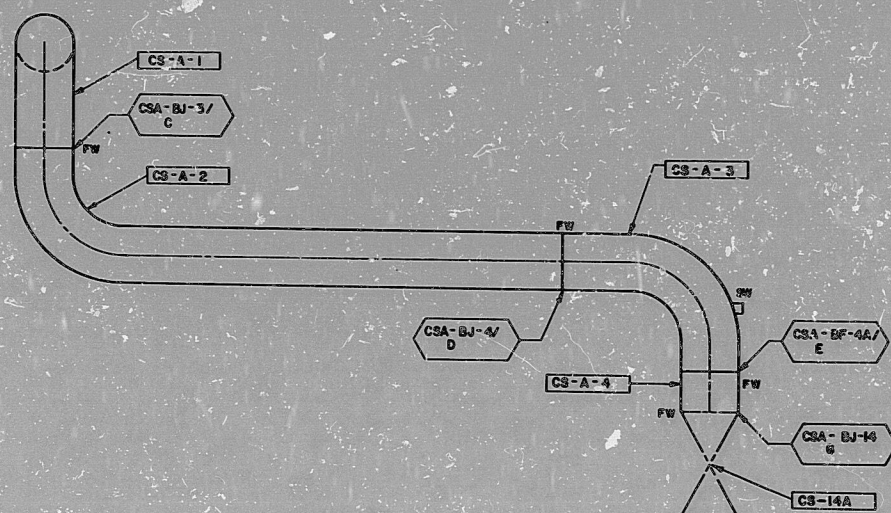
ELEVATION A-A
