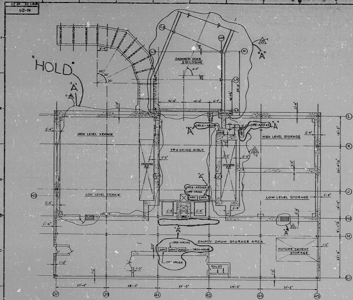
PLAN EL 397'-0"
