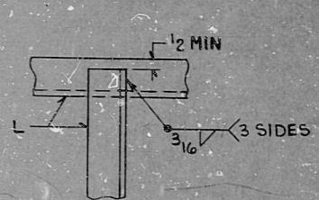
DET DJ
