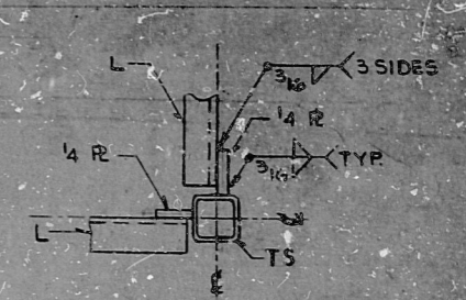
SECT DD
