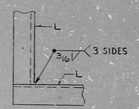
DET DH
