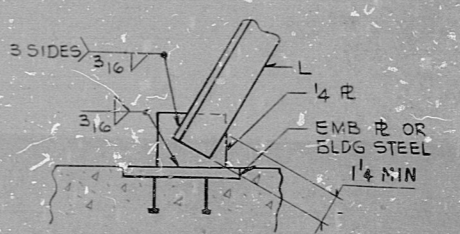
DET DL
