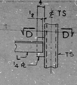
DET DD
