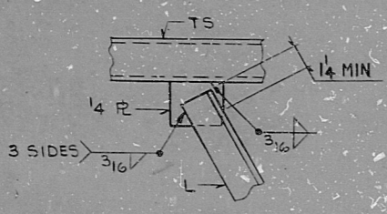
DET DE
