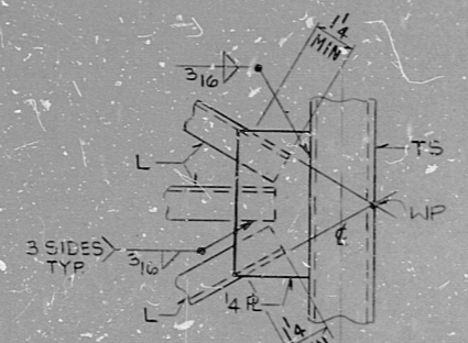
DET DF
