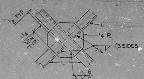
DET DC
