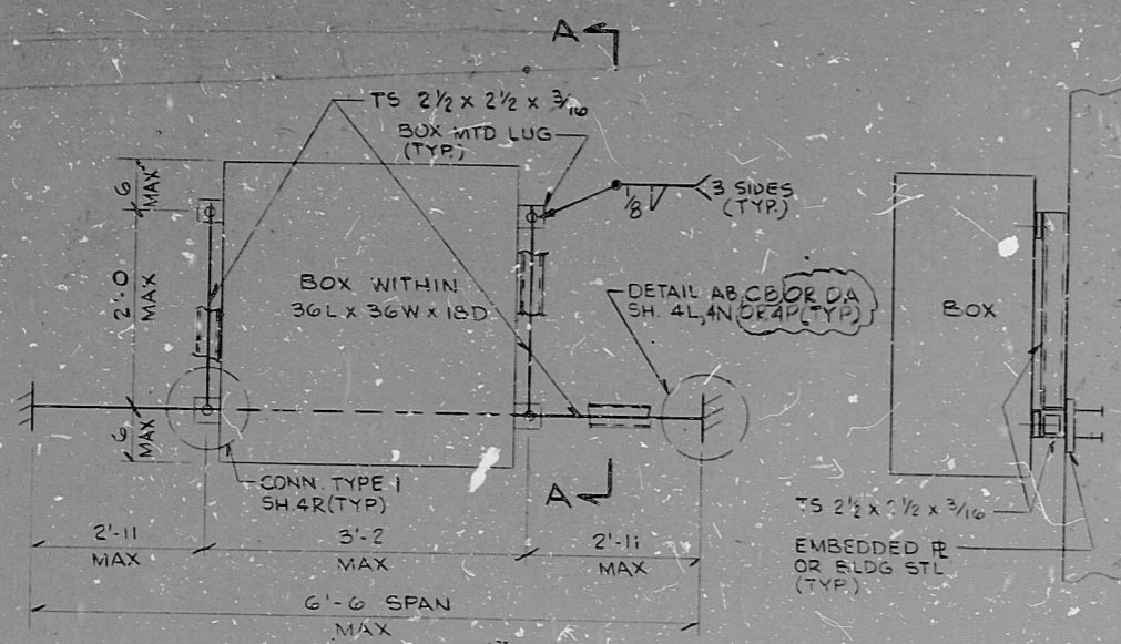
DETAIL 16A N.T.S.
