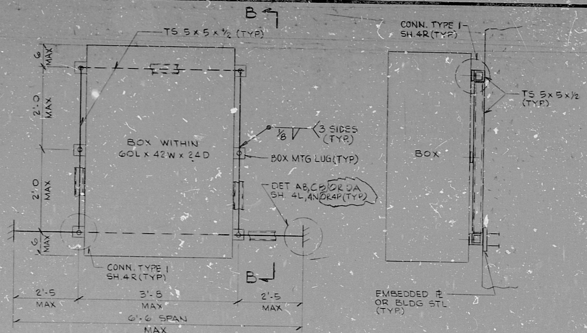
DETAIL 16B N.T.S.
