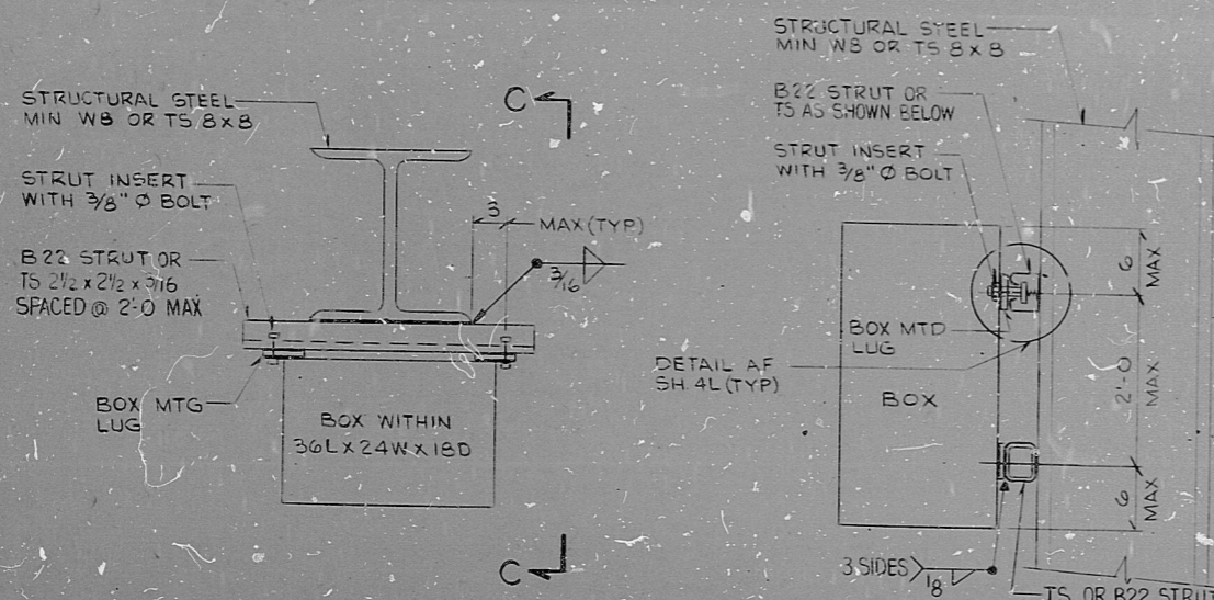
DETAIL 17A N.T.S.
