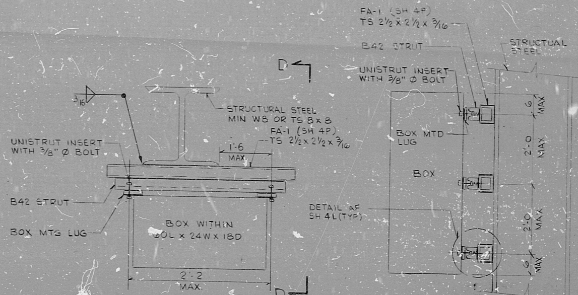
DETAIL 18A N.T.S.
