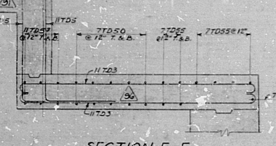
SECTION F-F Scale: 3/8"=1'-0"
