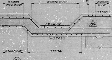
SECTION E-E Scale: 3/8"=1'-0"
