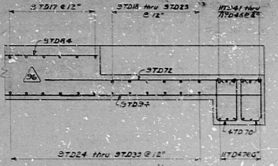
SECTION D-D Scale: 3/8"=1'-0"
