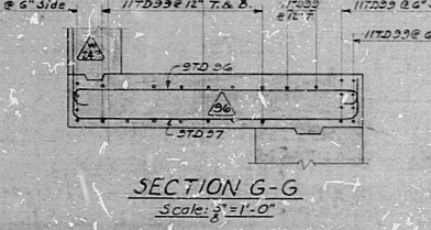
SECTION G-G Scale: 3/8"=1'-0"
