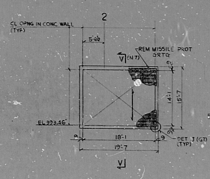
ELEV C (D17)
