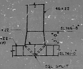
SECTION AA-AA SCALE: 1/4"=1'-0"
