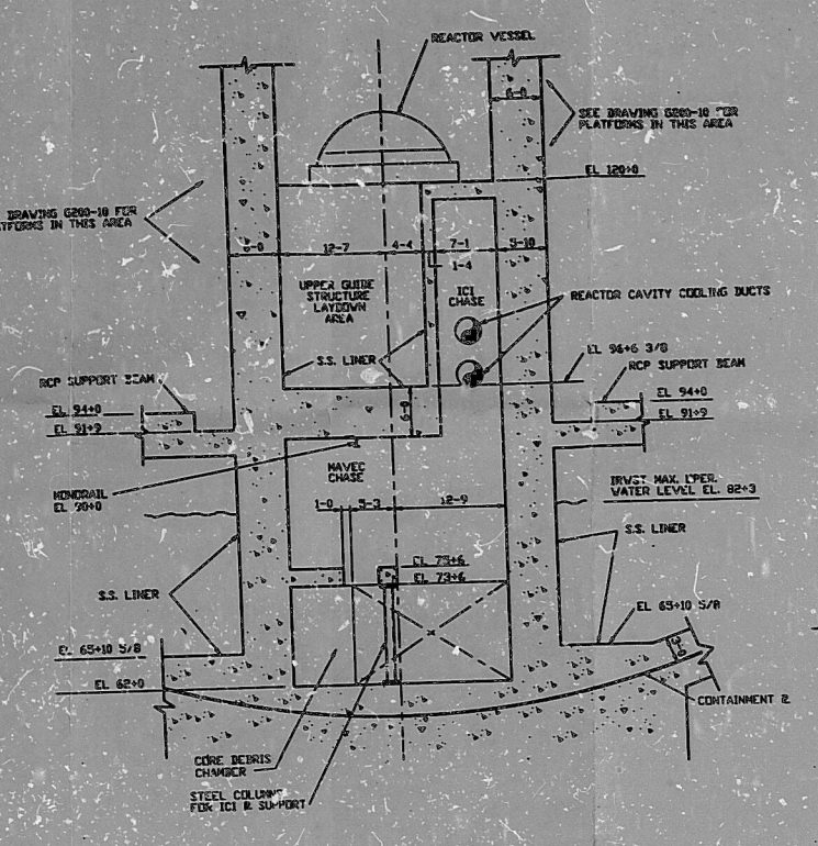
A SECTION THRU MAVEC CHASE
