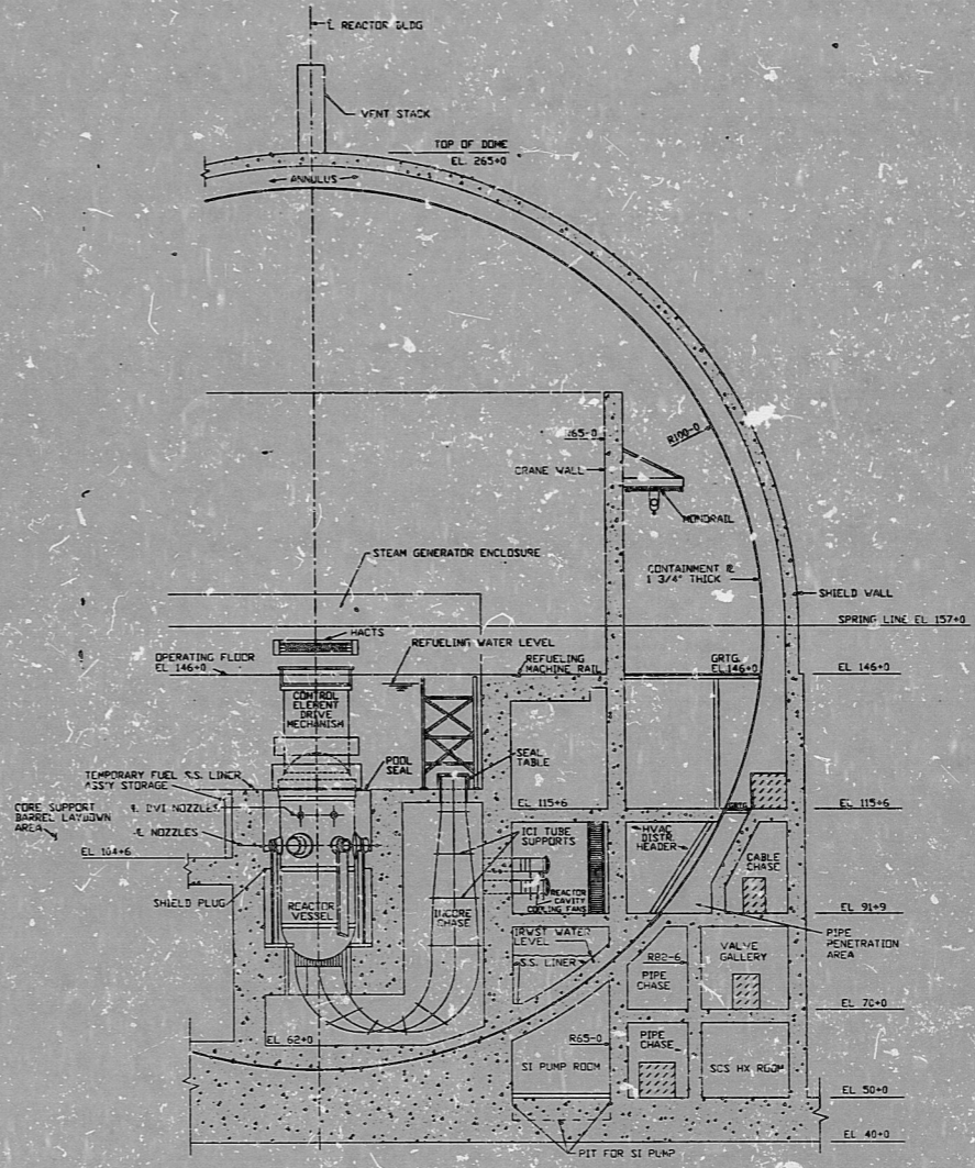
C SECTION THRU ICI CHASE GEO-11
