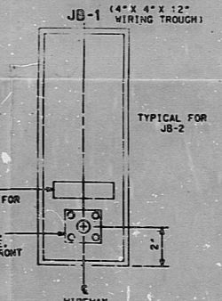
DETAIL 26 N.T.S.
