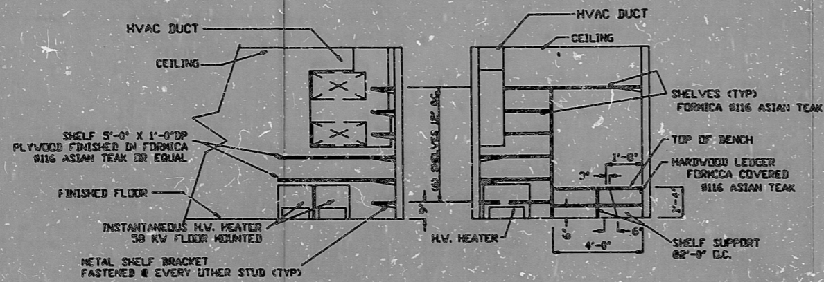
ELEVATION A-A
