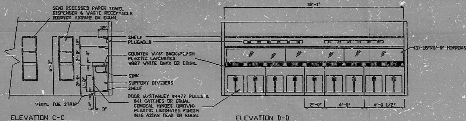
ELEVATION C-C
