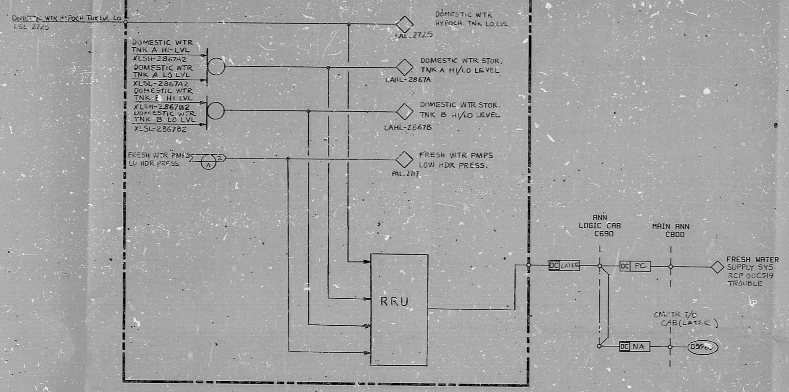
ALARM INPUTS
