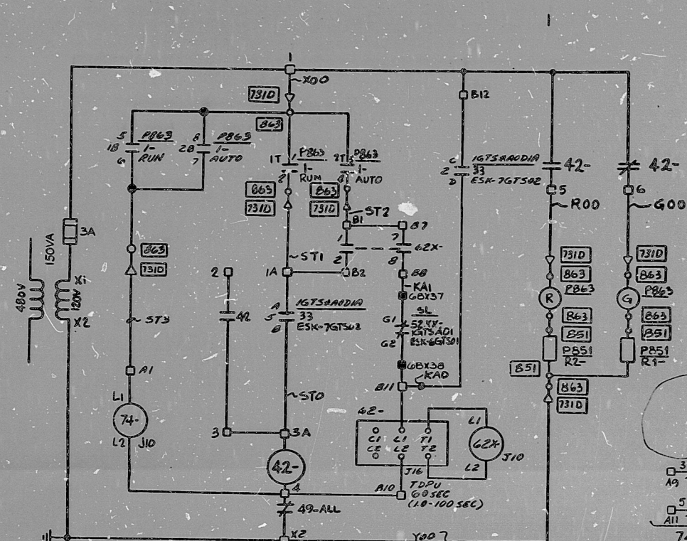
STBY GAS TRTMT DECAY HT REMOVAL FAN IGTS*FN2A CKT NO IGTS A03 LOCN. IEH5*MCC2C (RED)
