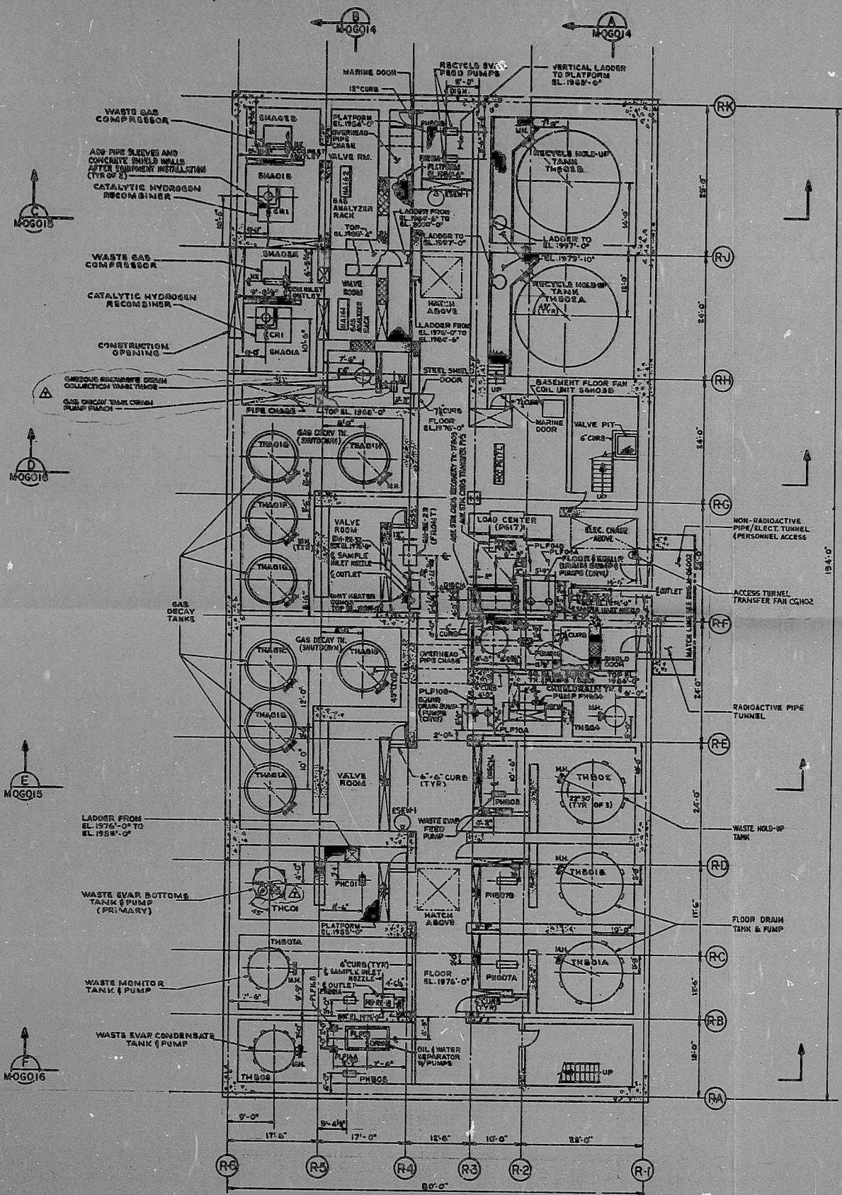
BASEMENT PLAN EL 1976'-0"
