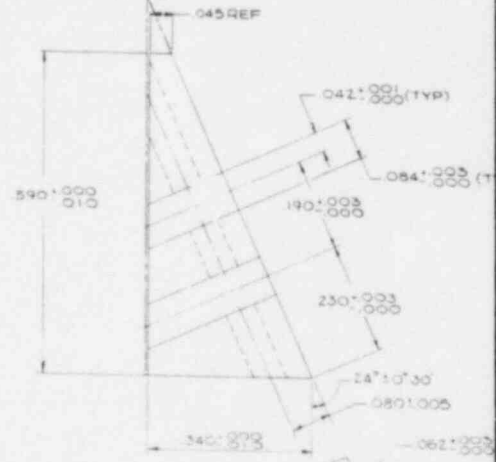
VIEW B-E SCALE 2:1
