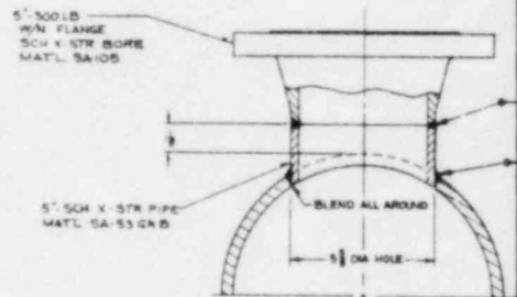
DETAIL A SCALE: 1/2
