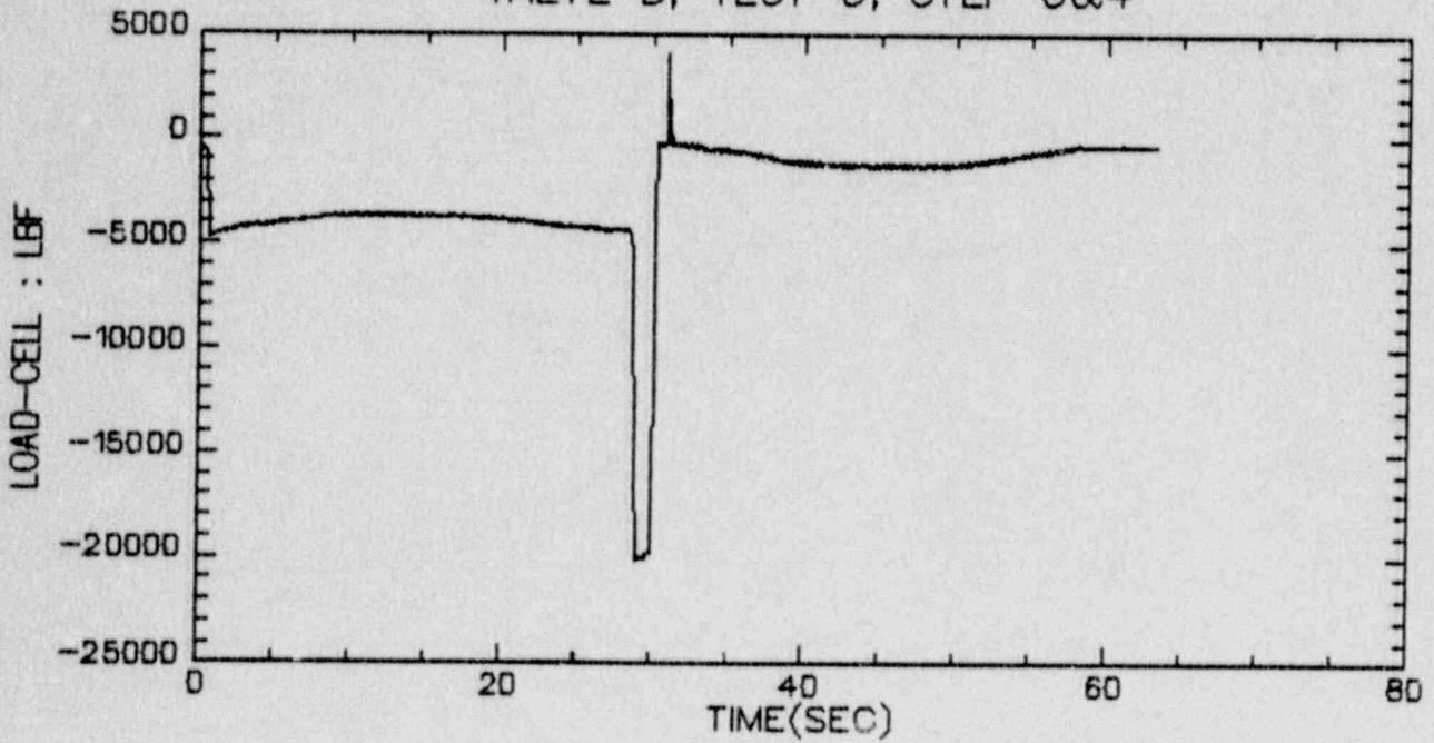
VALVE B, TEST 5, STEP 3&4
