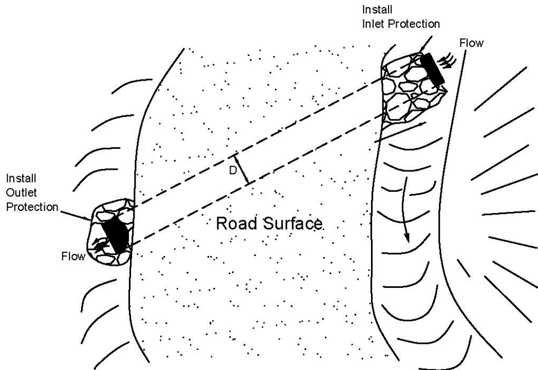
A. PLAN
