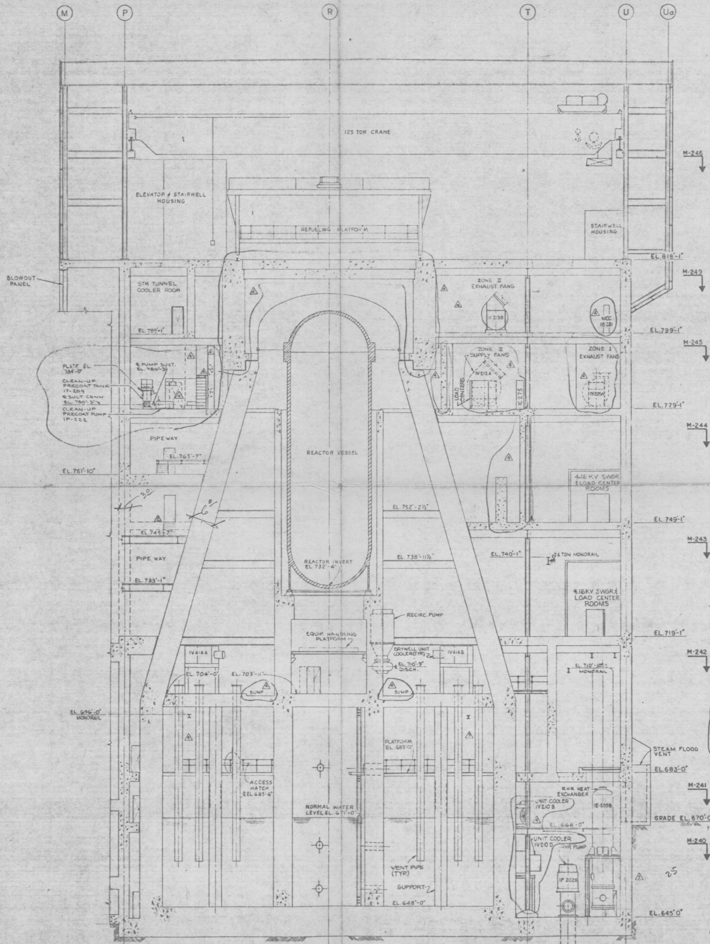
EQUIP. LOC. RA. SECTION A-A
