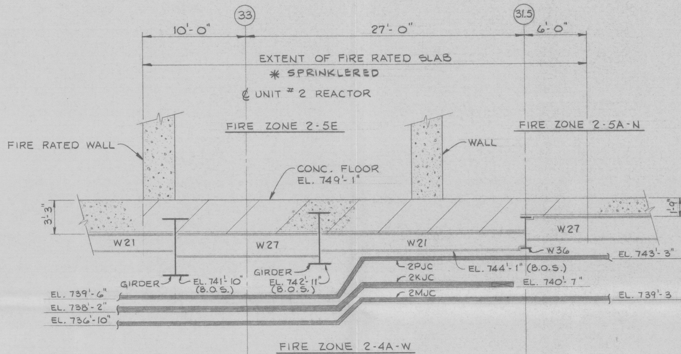
SECTION A-A SCALE: 3/16" = 1'-0"
