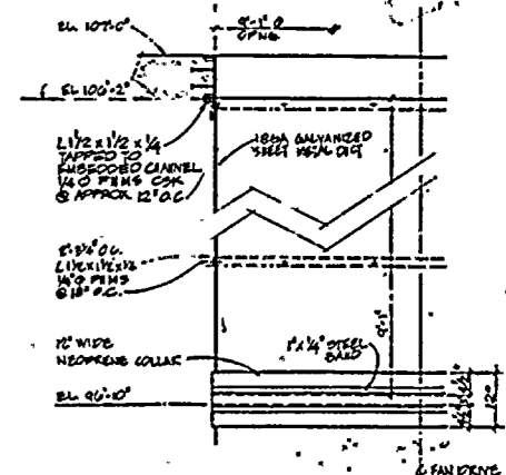
ⓐ DIESEL ENGINE RADIATOR FAN EXH. DET.
