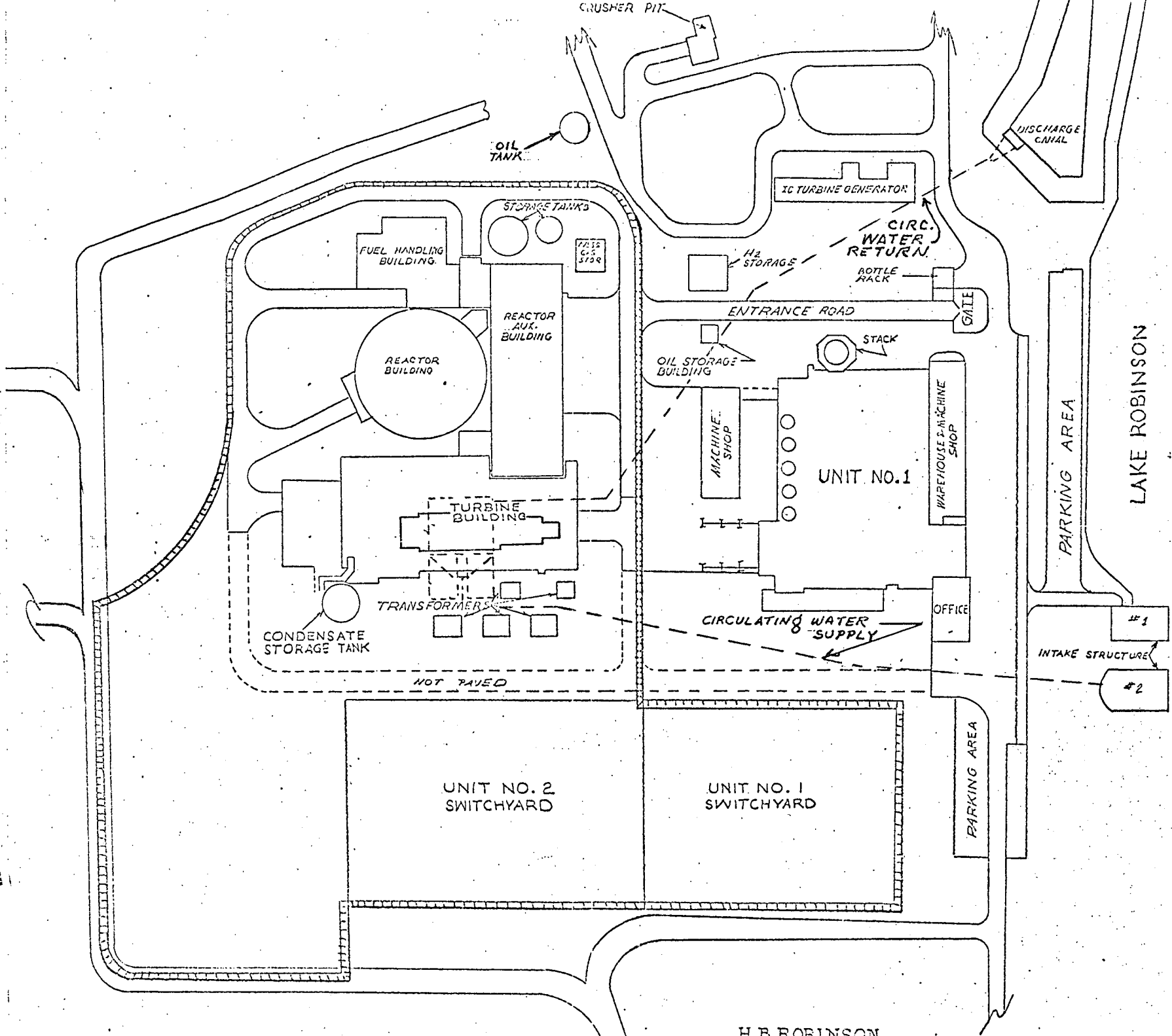
H.B. ROBINSON PLOT PLAN
