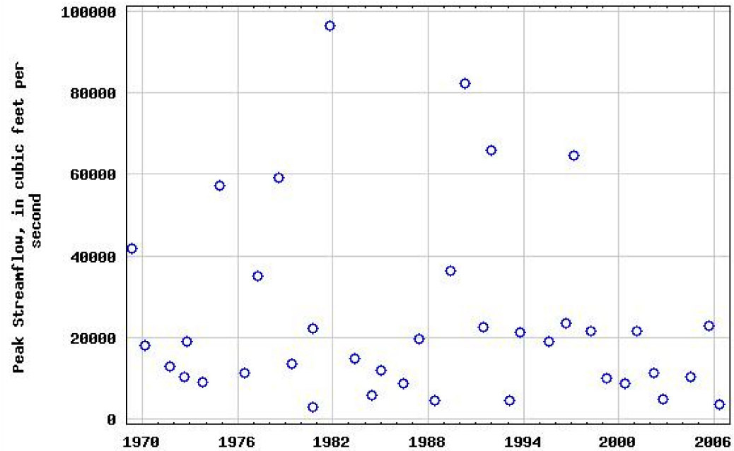
USGS 08090800 Brazos Rv nr Dennis, TX
