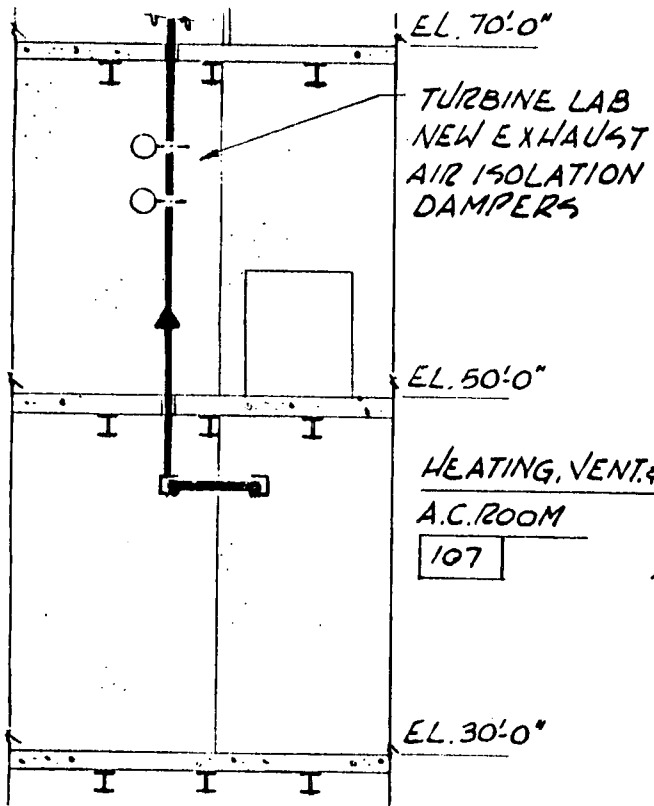
SECTION-A
