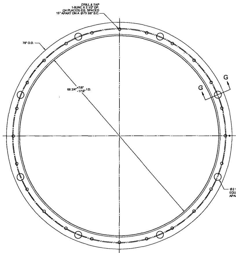
TOP FLANGE
