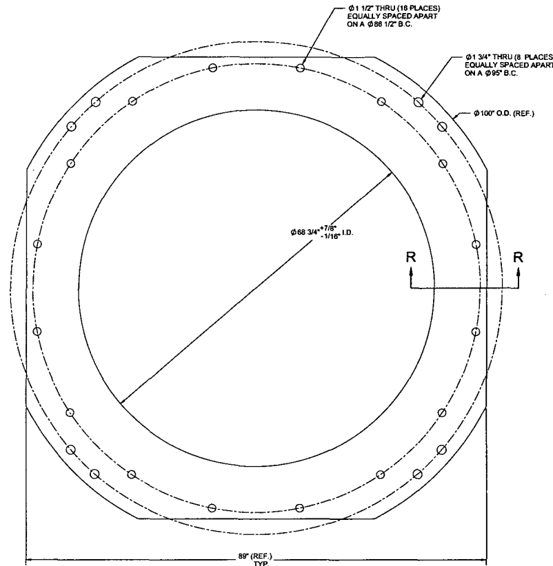
BOTTOM FLANGE
