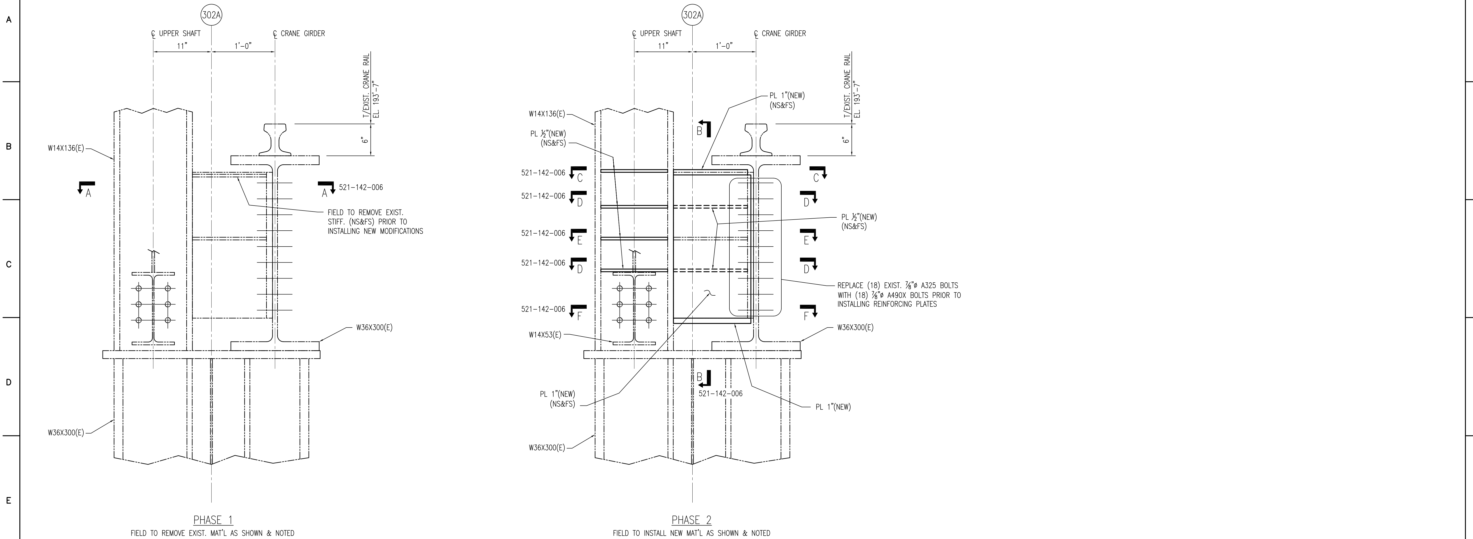
DETAIL A SCALE: 1 1/2"=1'-0" DWG. S-521-102
