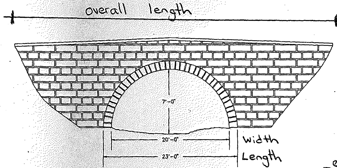
ELEVATION
