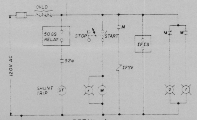
CONTROL CKT SCHEMATIC FOR MFAN-001 & MFAN-002
