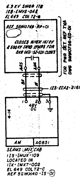
161KV & 500KV SWYD XFMR FDR BKR SEAMS ALARM
