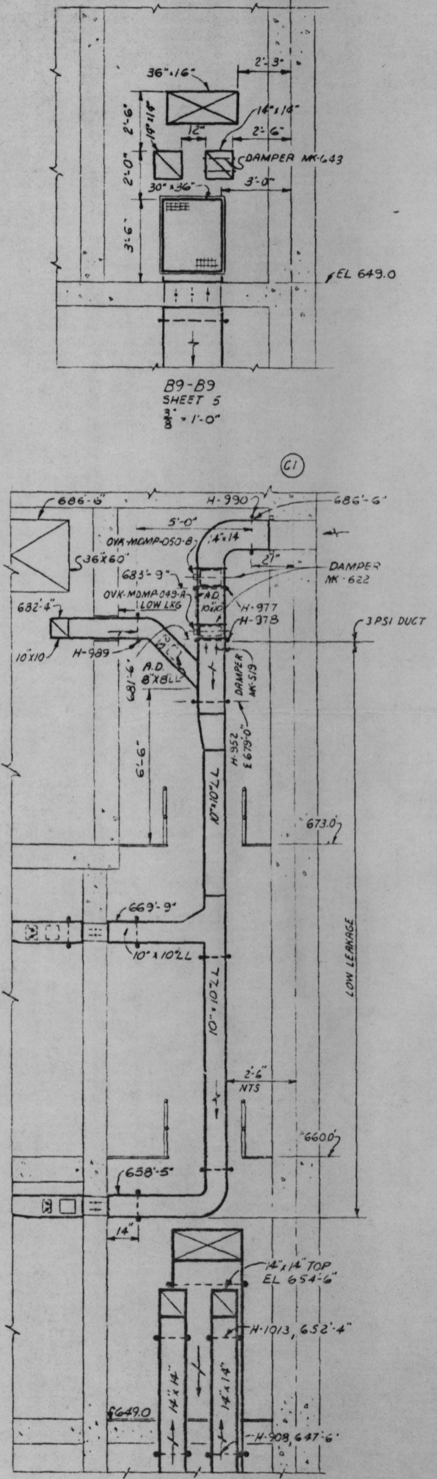
C9-C9 SHEETS 5 & 6 3/4\"/>
