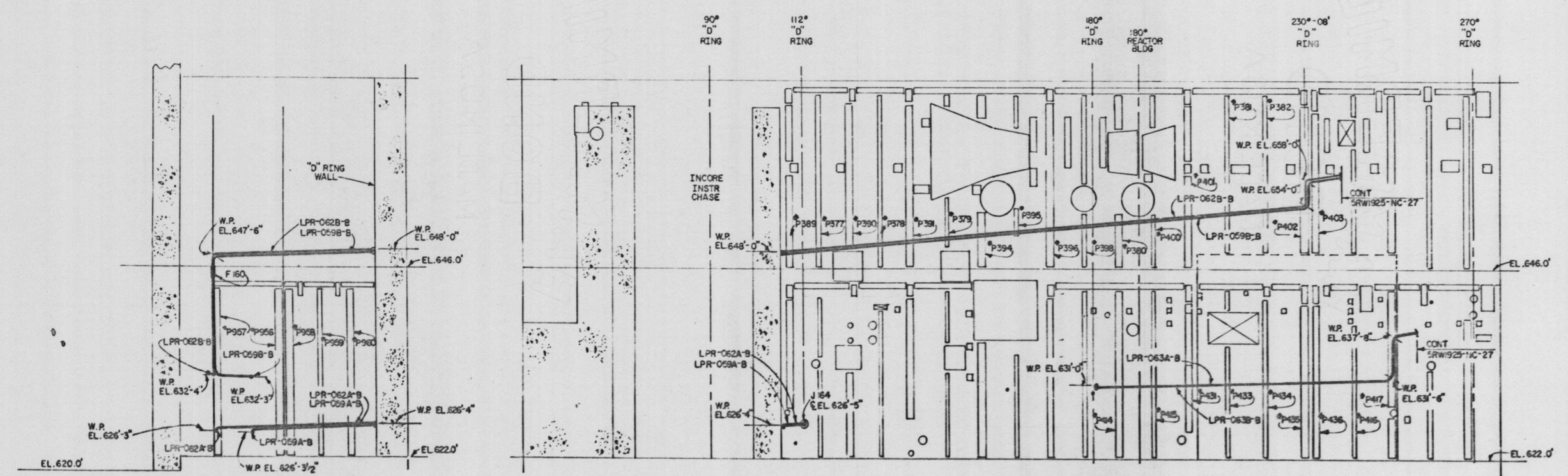
D26-D26 SCALE: 1/8" = 1'-0" SHEET 23 & 24
