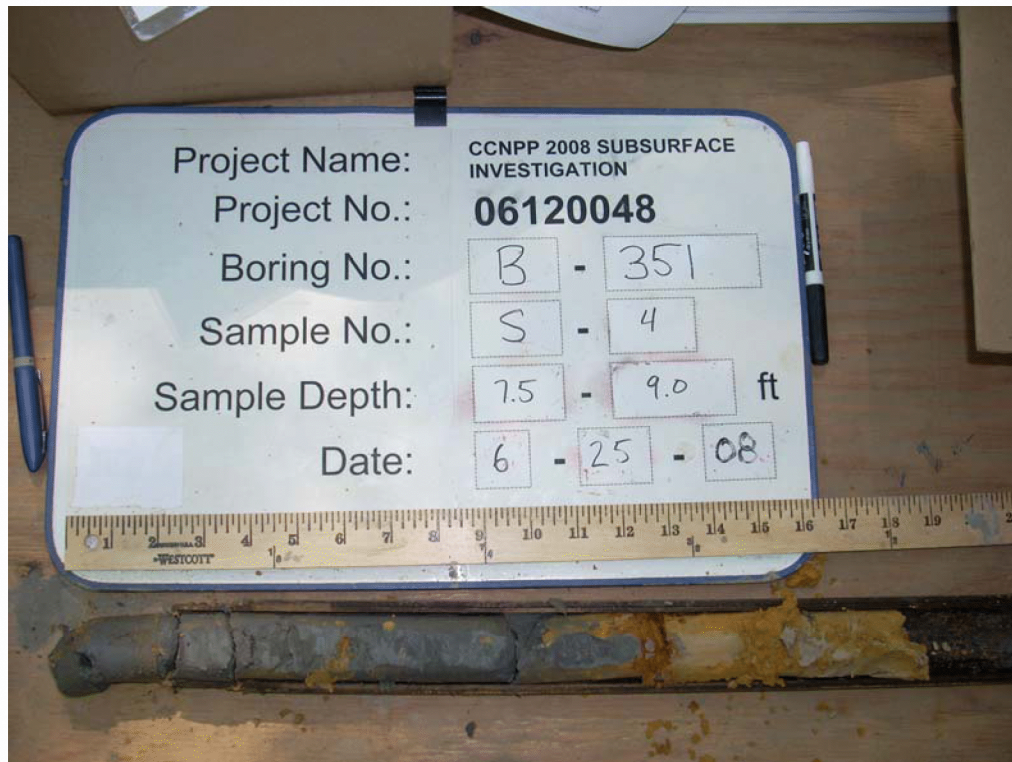
B-351; S-4 7.25 - 9.0 ft
