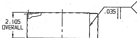
CAP WRAPPER ELEVATION
