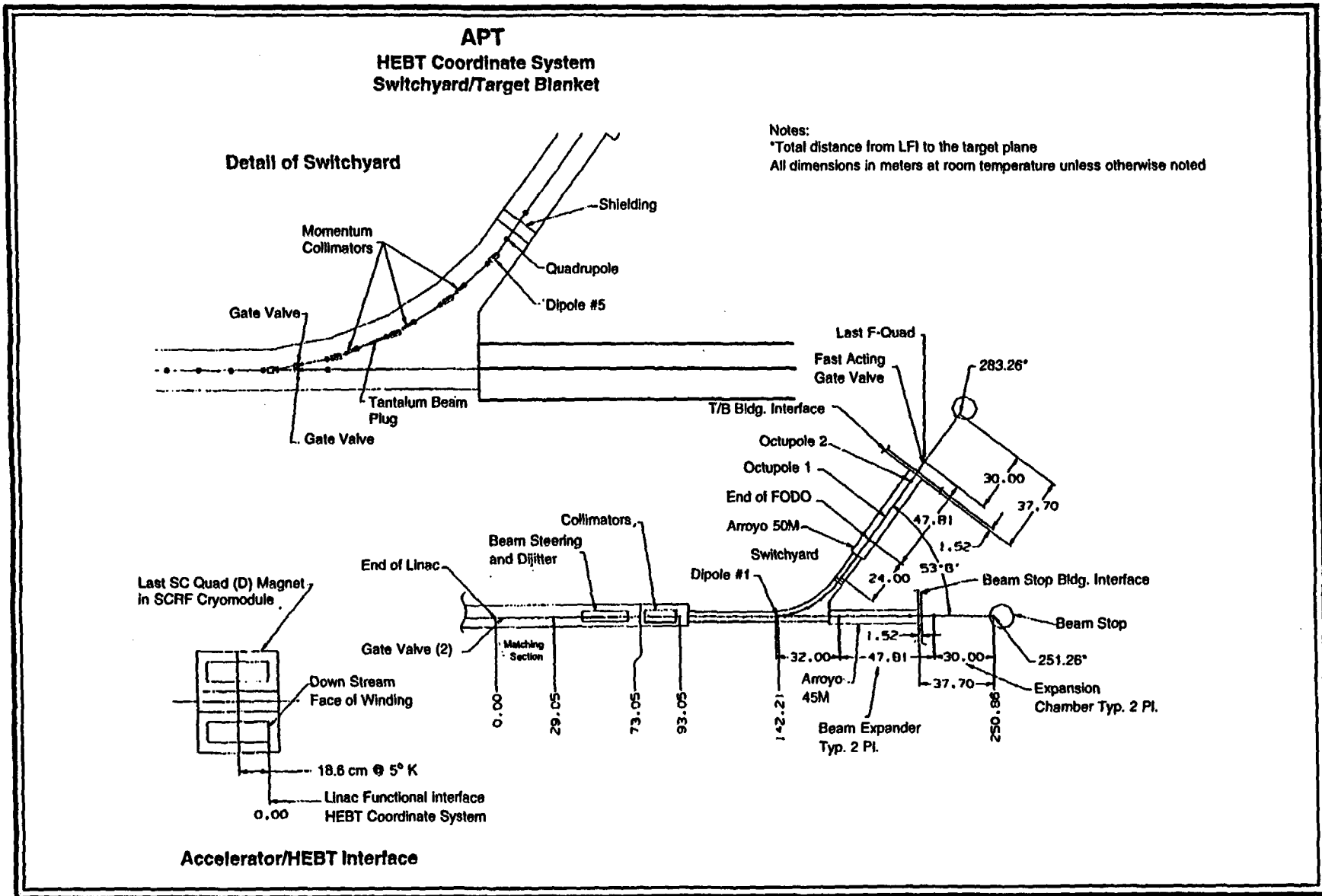
Figure A-8. Switchyard (LANL 1997).
