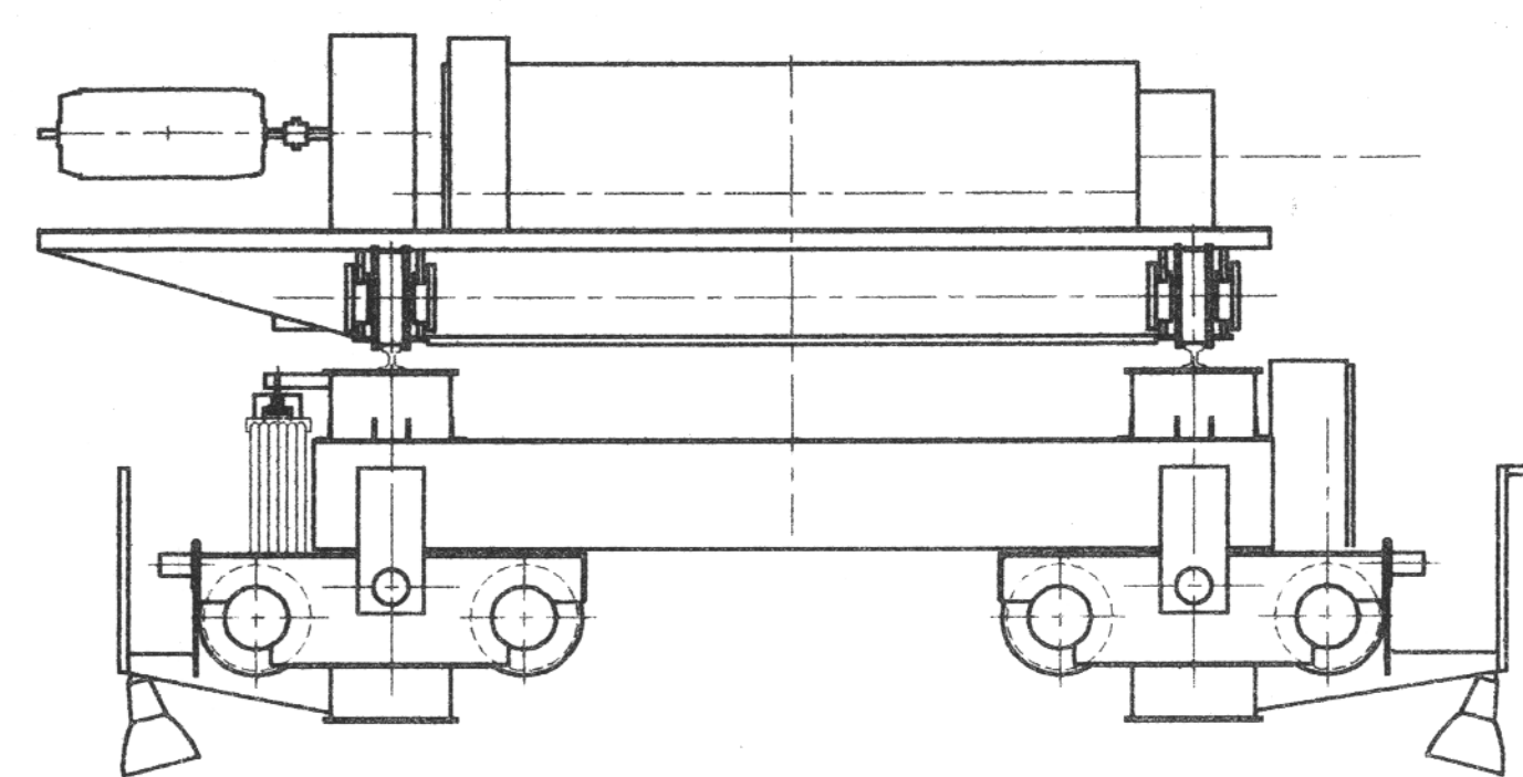
VIEW A-A
