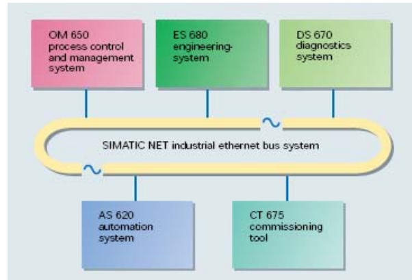
Fig. 2.10. TELEPERM XP subsystems.
